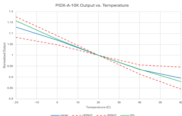
Fig. 3 PIDX-A-10K 灵敏度温度特性
