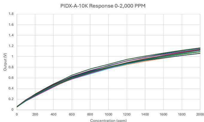
Fig. 2 PIDX-A-10K 响应 (0-2000 ppm)
